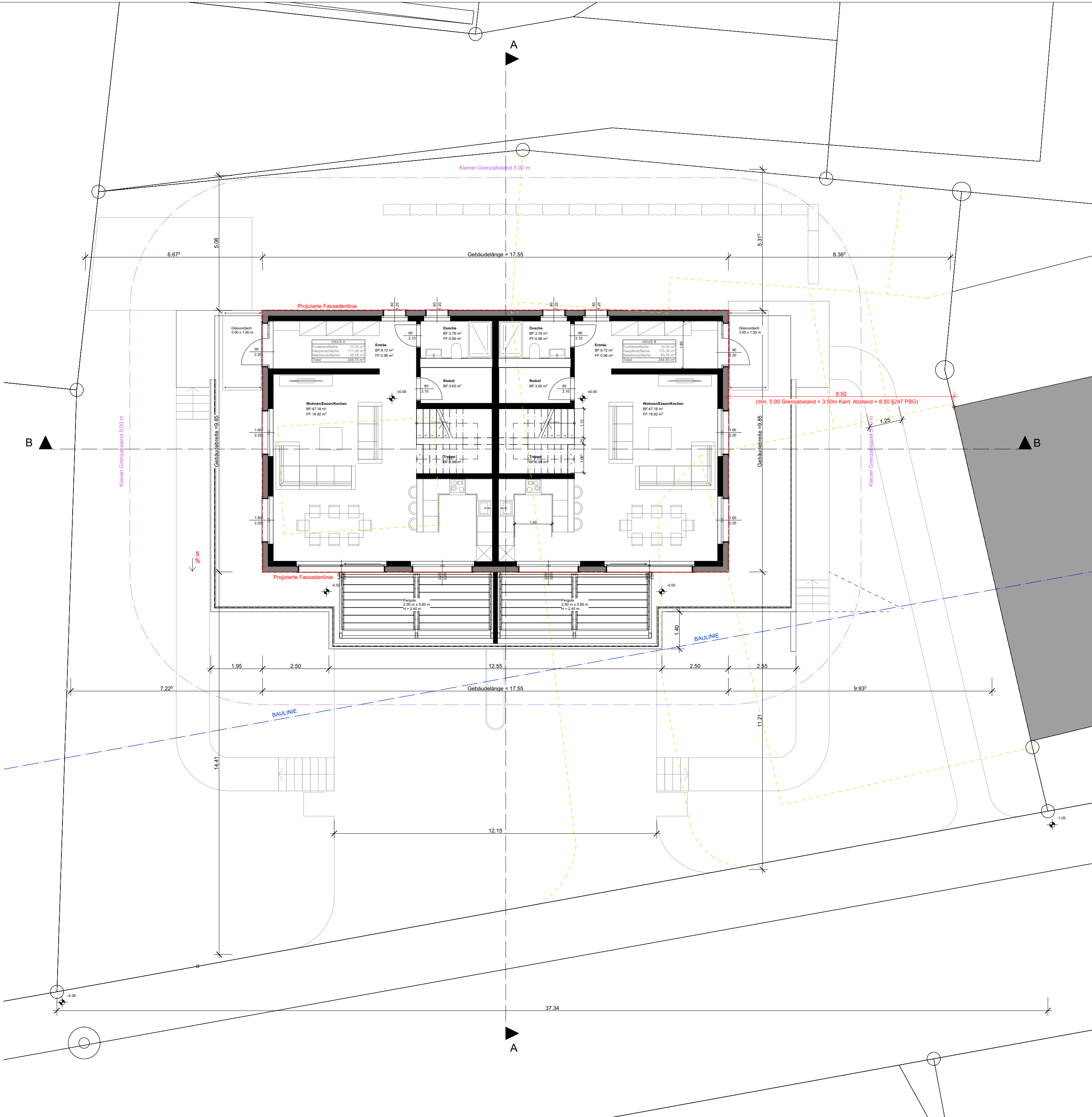
Erdgeschoss / Umgebung
