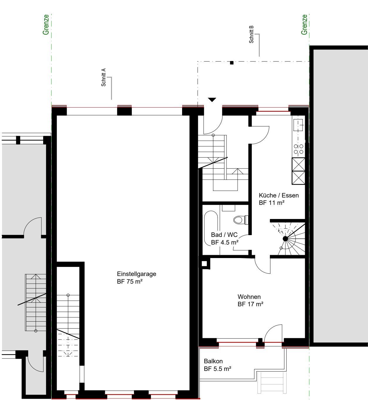
Erdgeschoss
