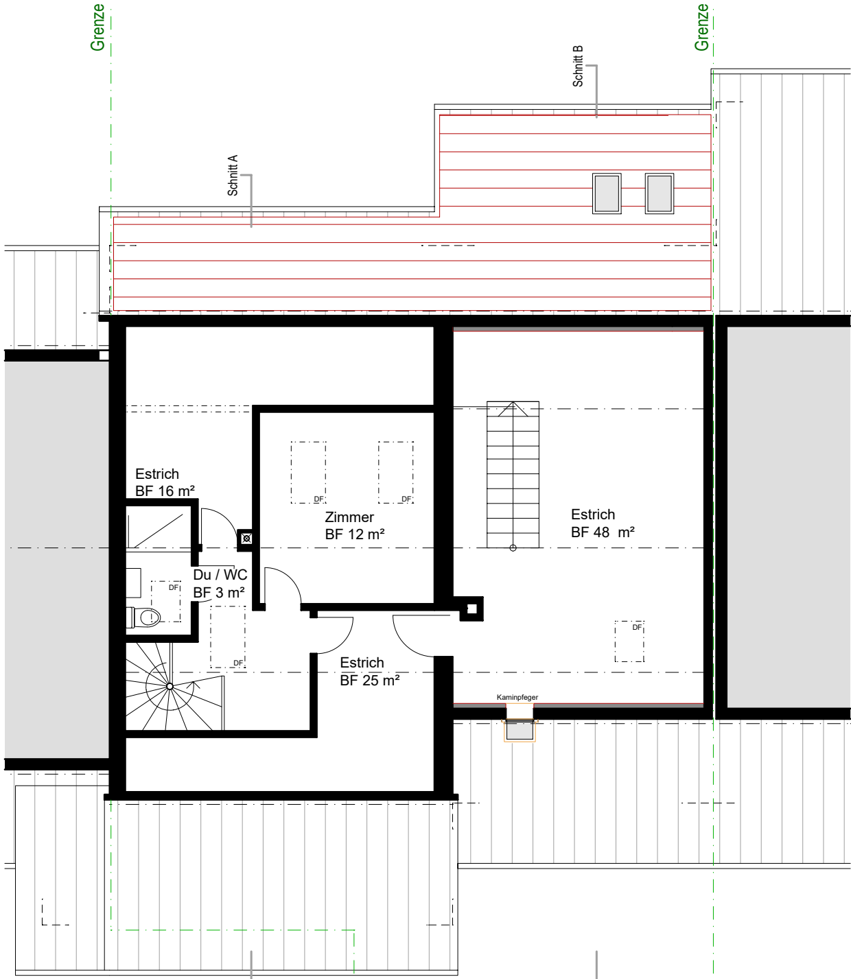
Dachgeschoss
