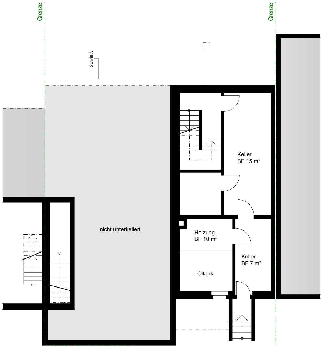
Untergeschoss
