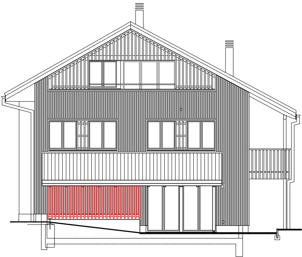
SÜDFASSADE
