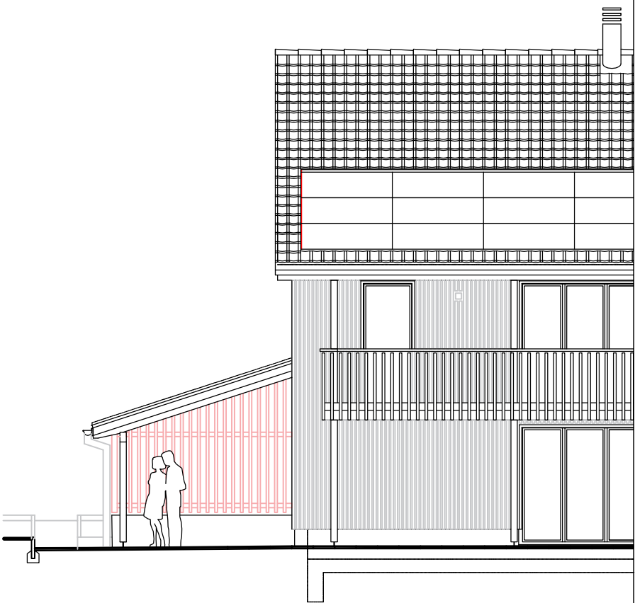
OSTFASSADE
