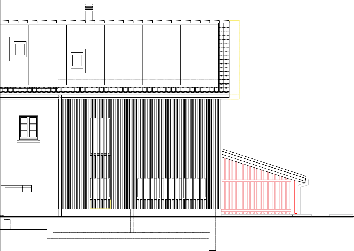
WESTFASSADE
