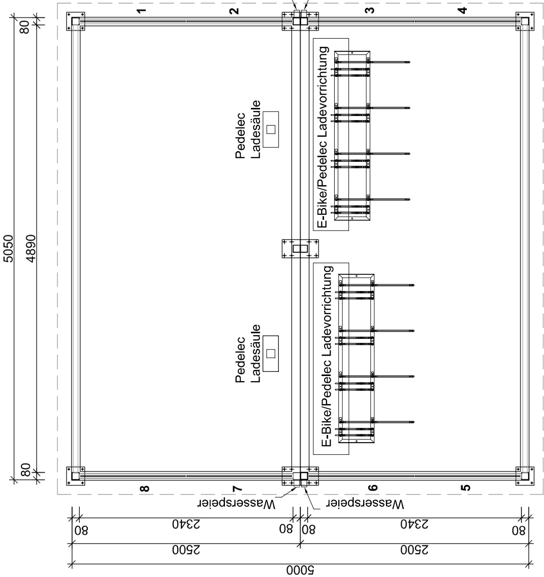
Grundriss
