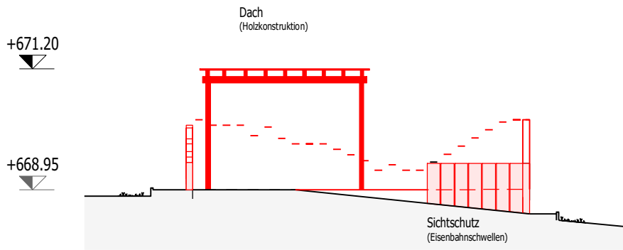
Westfassade
