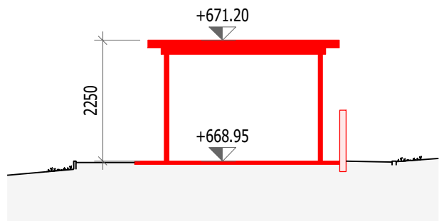
Schnitt A-A
