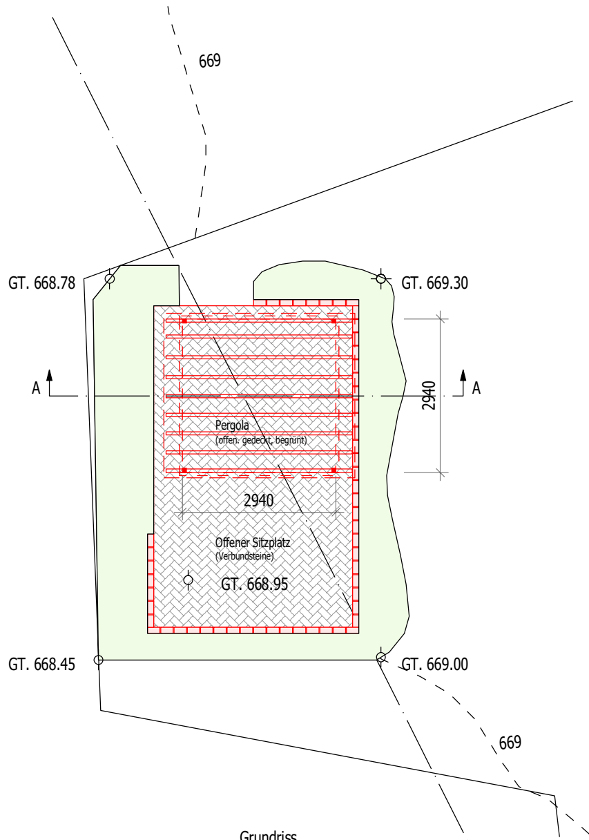
Grundriss
