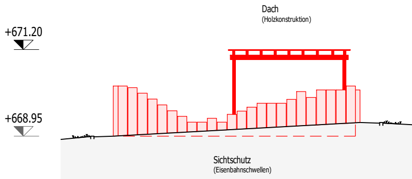
Ostfassade
