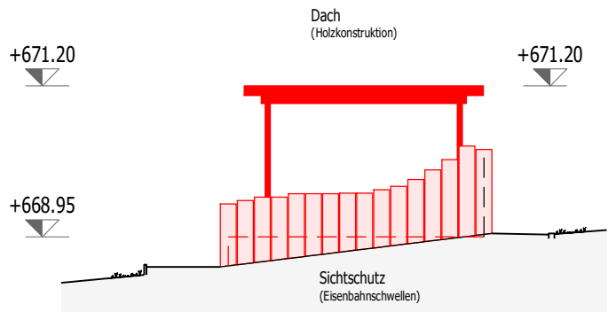
Südfassade
