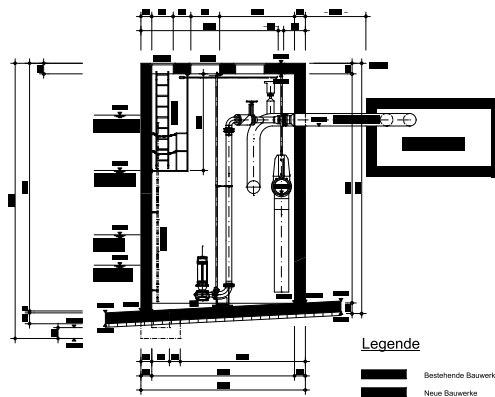
Schnitt A-A 1:50
