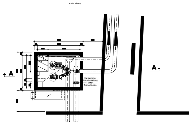
Grundriss 1:50
