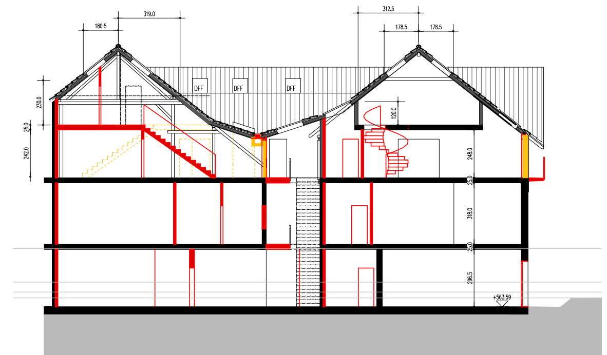
Schnitt D-D
