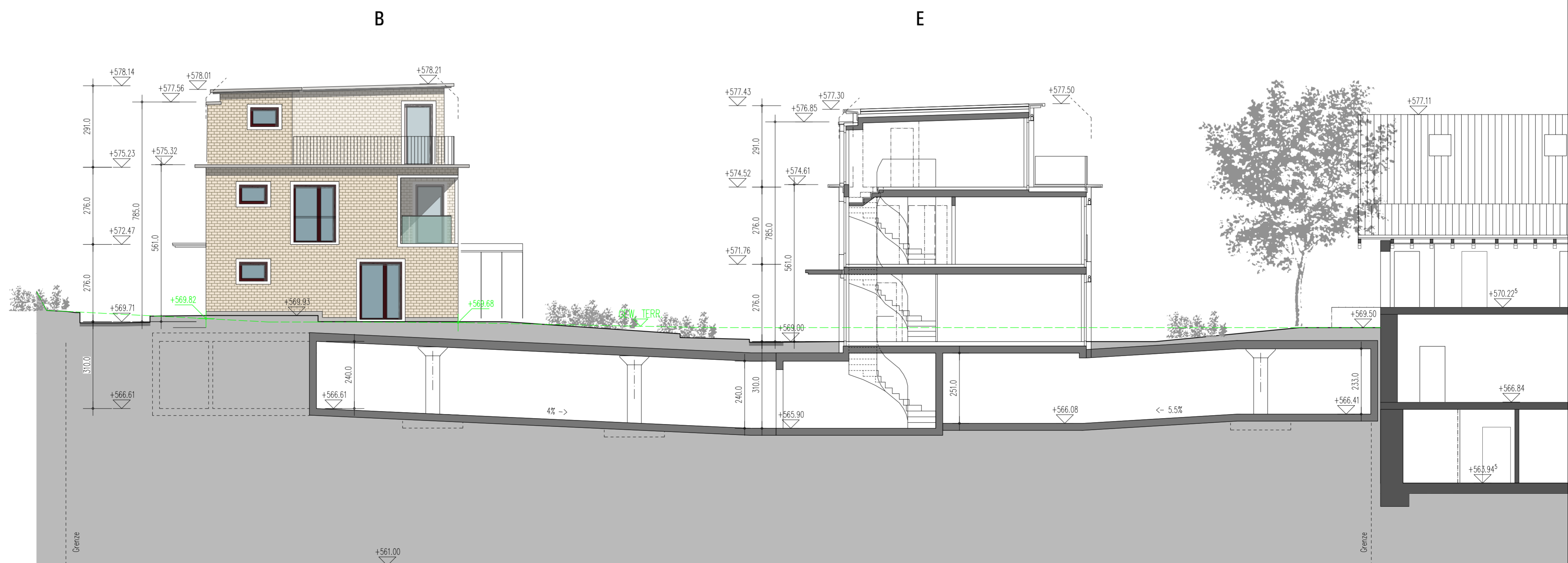
Westfassade / Schnitt 06
