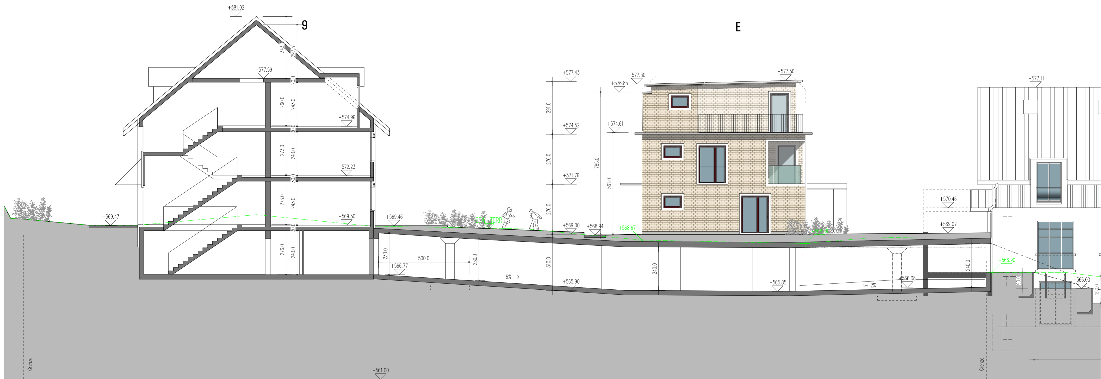
Westfassade / Schnitt 08
