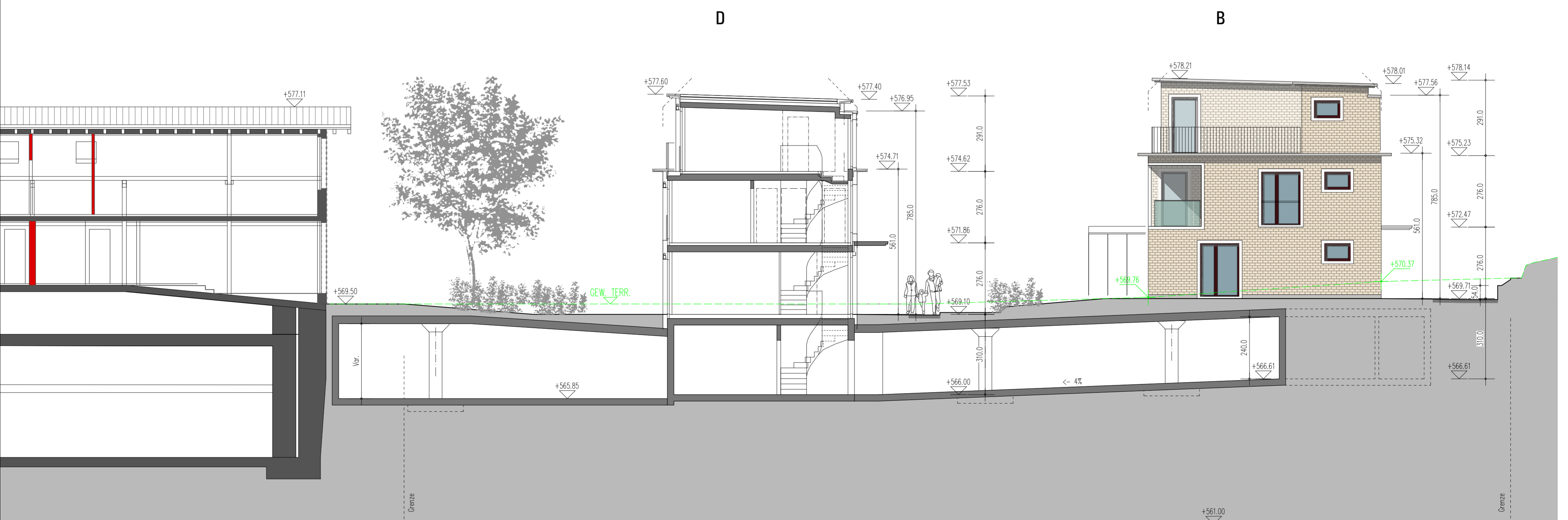
Ostfassade / Schnitt 05
