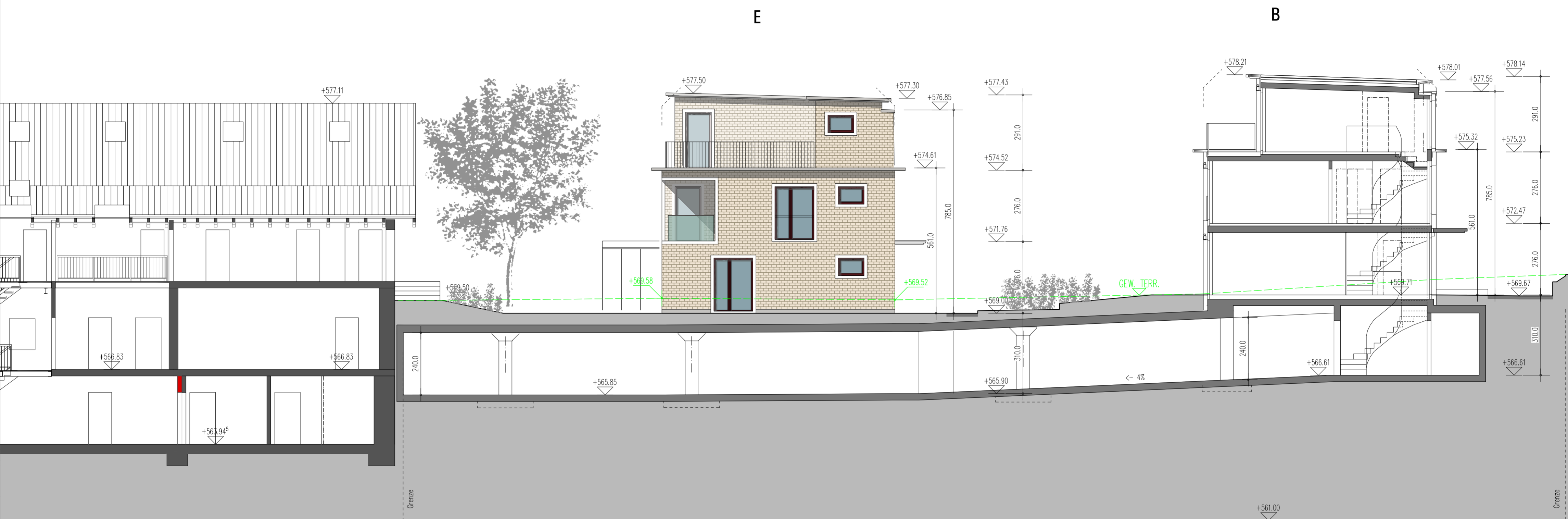
Ostfassade / Schnitt 07
