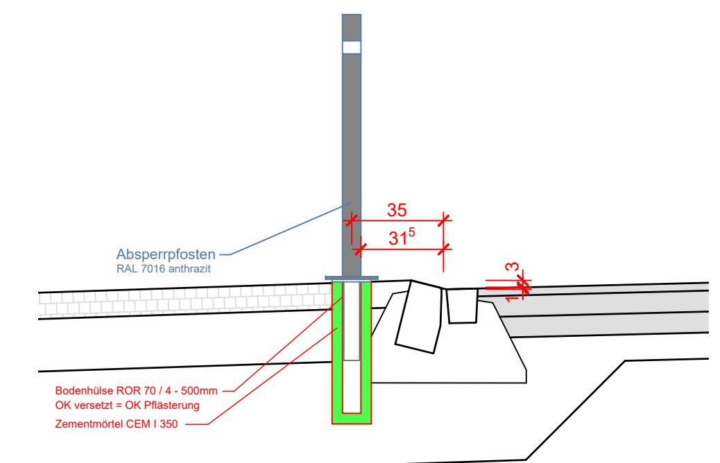
Detail Absperrpfosten, 1 : 20
